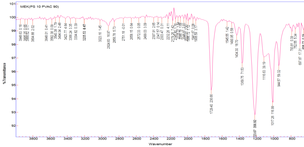
Fig.1 (a): FTIR PS (10) + PVAc (90) (MEK)
